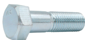
Pernos Hexagonales- diámetro 1.1/4 - grado 2 - Zincado
